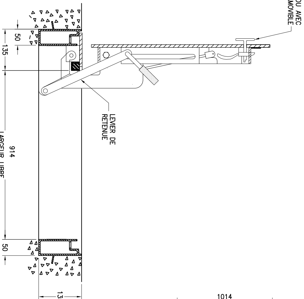
COUPE A-A ECH. P.A.E.
